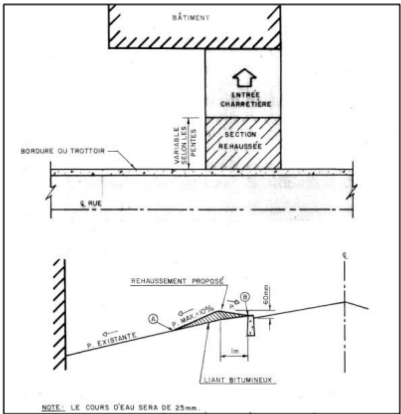
Illustration 17.1 Rehaussement d'une allée d'accès
